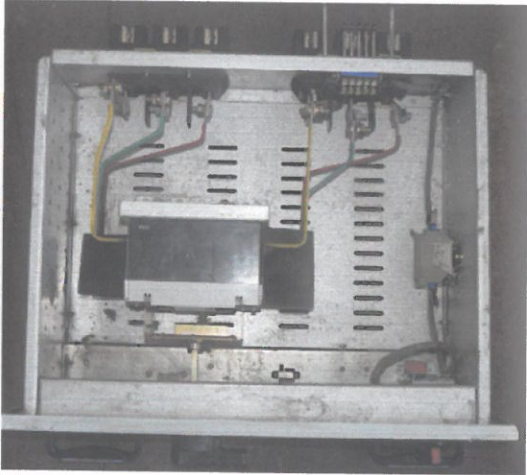
1 单元内部结构:
